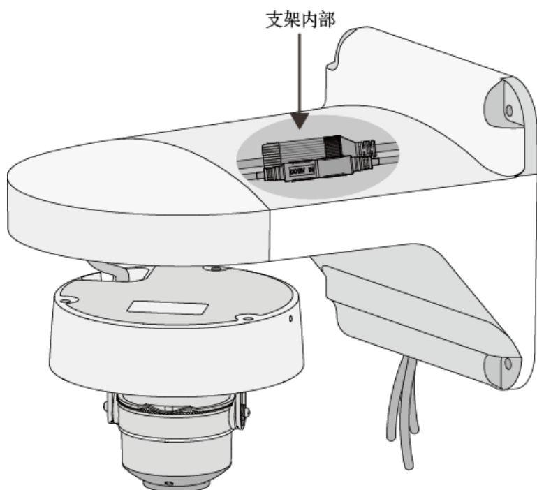
图2-11 支架内走线
