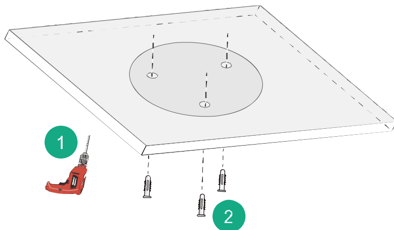
图2-8 安装面开孔示意图
